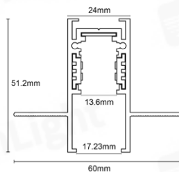
HS-15D 暗裝軌道條
